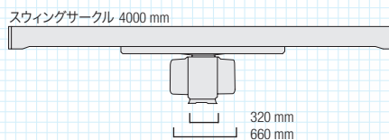
NKE-1139 3ユニット構成 質量：165kg
