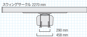
NKE-1129-7 3ユニット構成 質量：51kg
