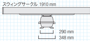
NKE-2103-6 質量：40kg
