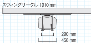
NKE-1125-6 質量：55kg
