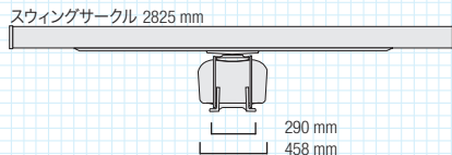
NKE-1125-9 質量：60kg
