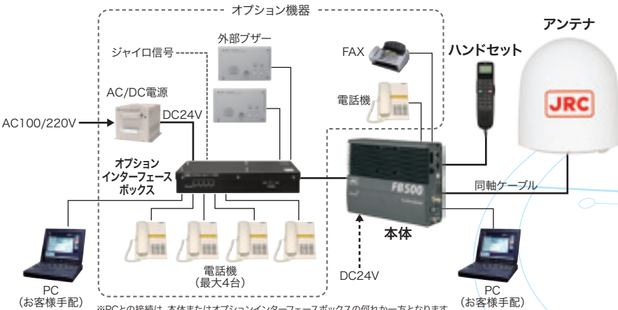
相互系統図
