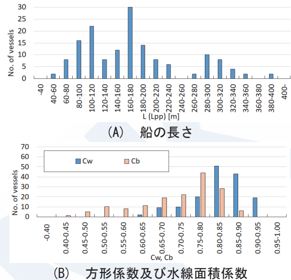
図2 数値解析対象船のヒストグラム
