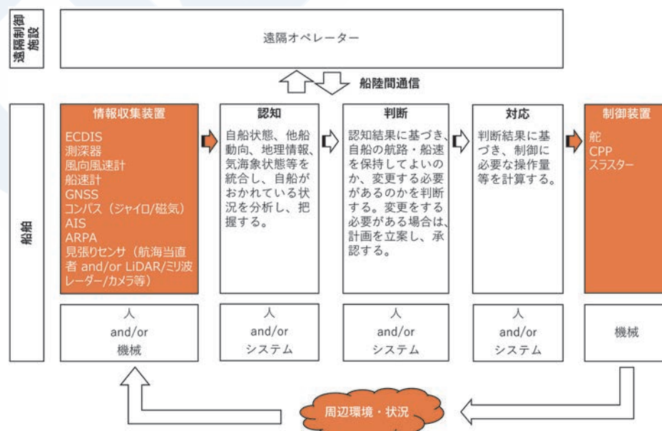
図5 操船業務の自動化・遠隔化のイメージ
