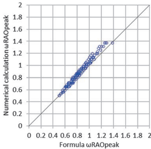
図10 式(21)と数値解析結果のHeave加速度の \omega_{RAOpeak} の比較
