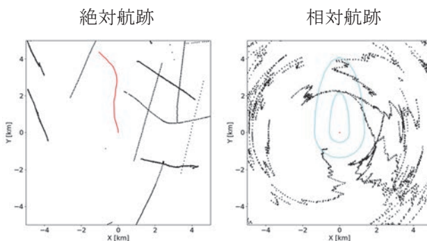
図11 AIによる自動操船結果 (バンパー内に相手船が存在する状況から開始)
