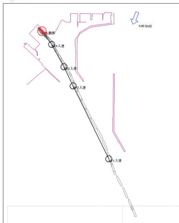
図11 実証試験航跡
