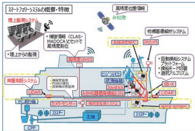
図1 スマートフェリーシステム装備配置概要
