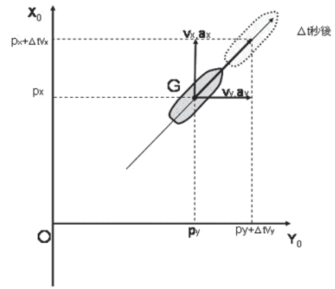
図5 航法フィルタにおける座標系
